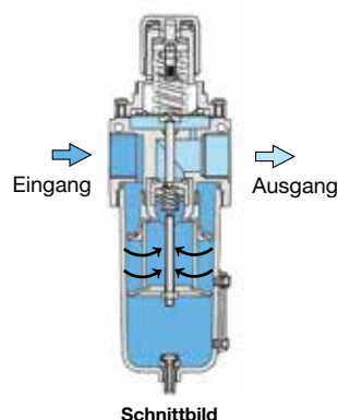
Schnittbild
